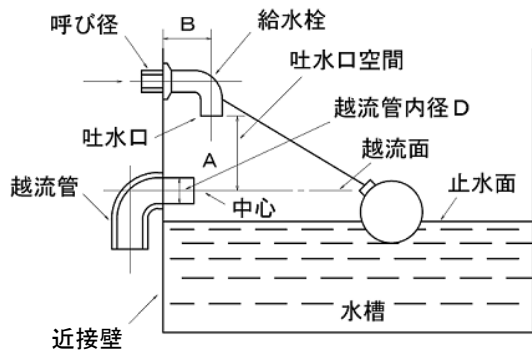
(1) 越流管（横取出し）
