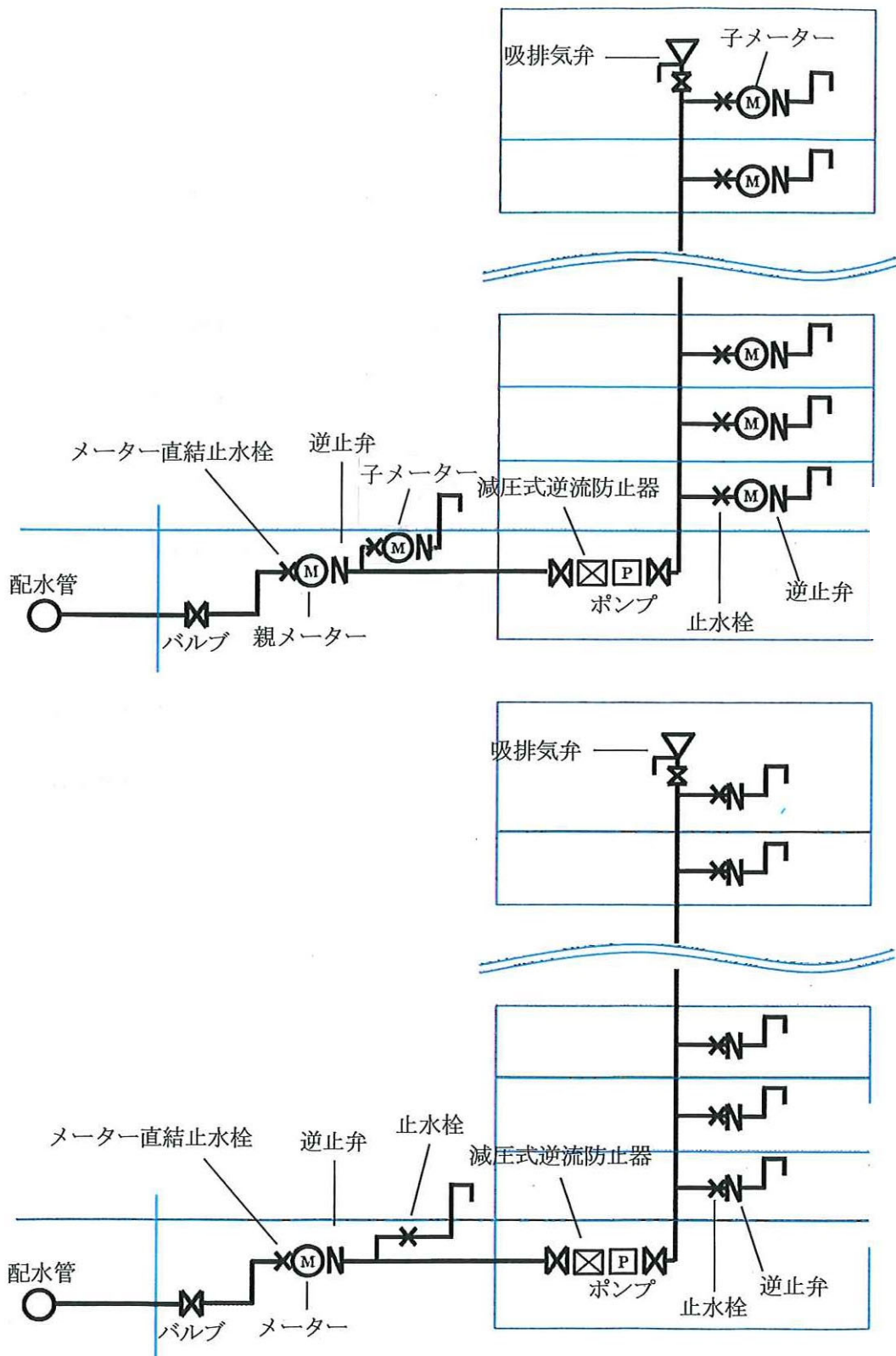
(2) 直結増圧式概念図
