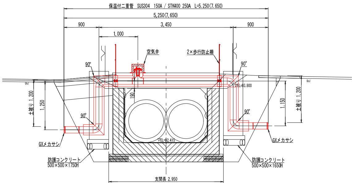
側面図(A-A) S=1:60
