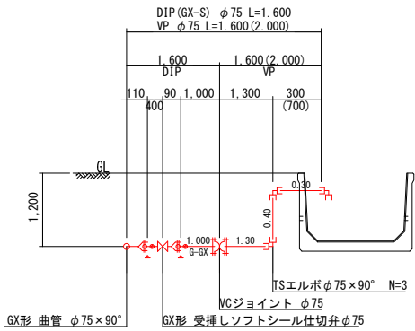
A-A断面図
