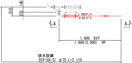
排水設備詳細図
