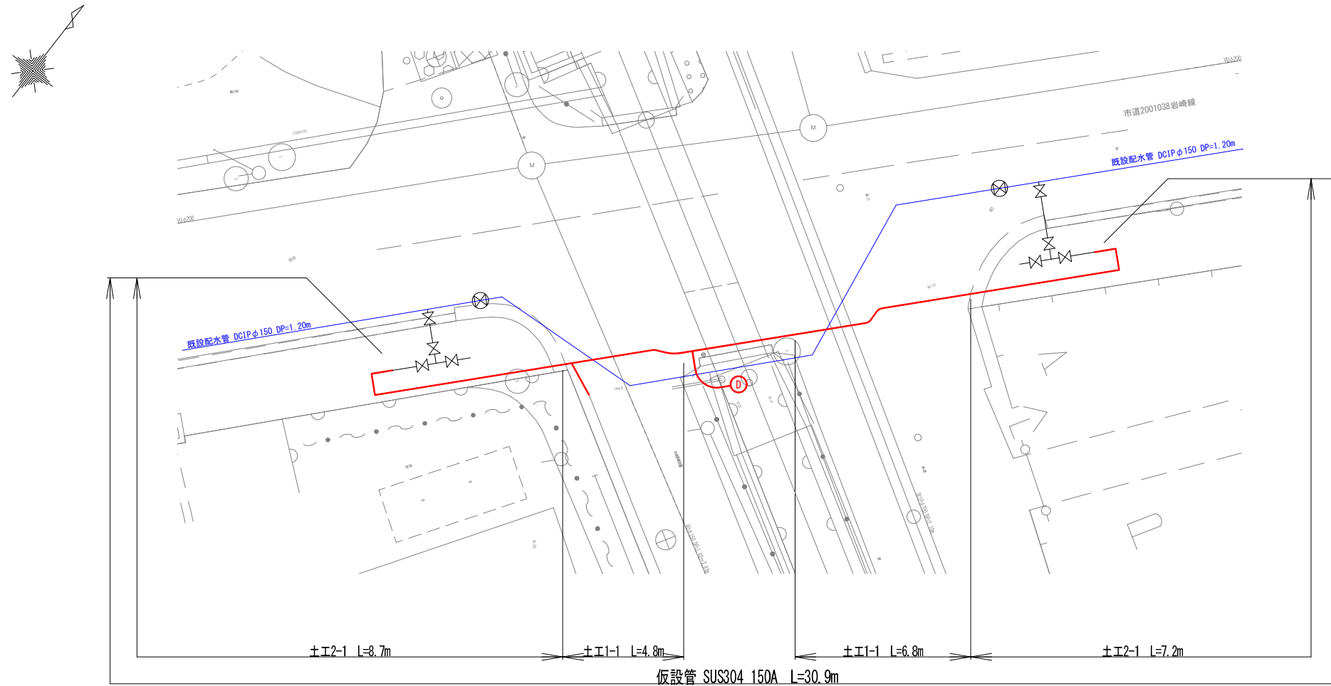
平面图 S=1:200
