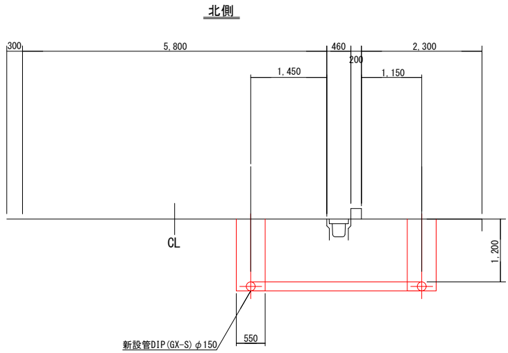
横断面 S=1:100
