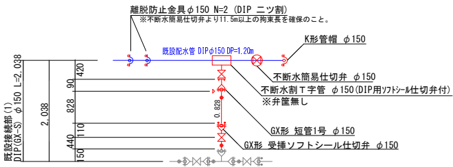
既設接続部(1)
