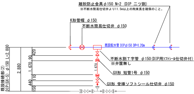
既設接続部(2)
