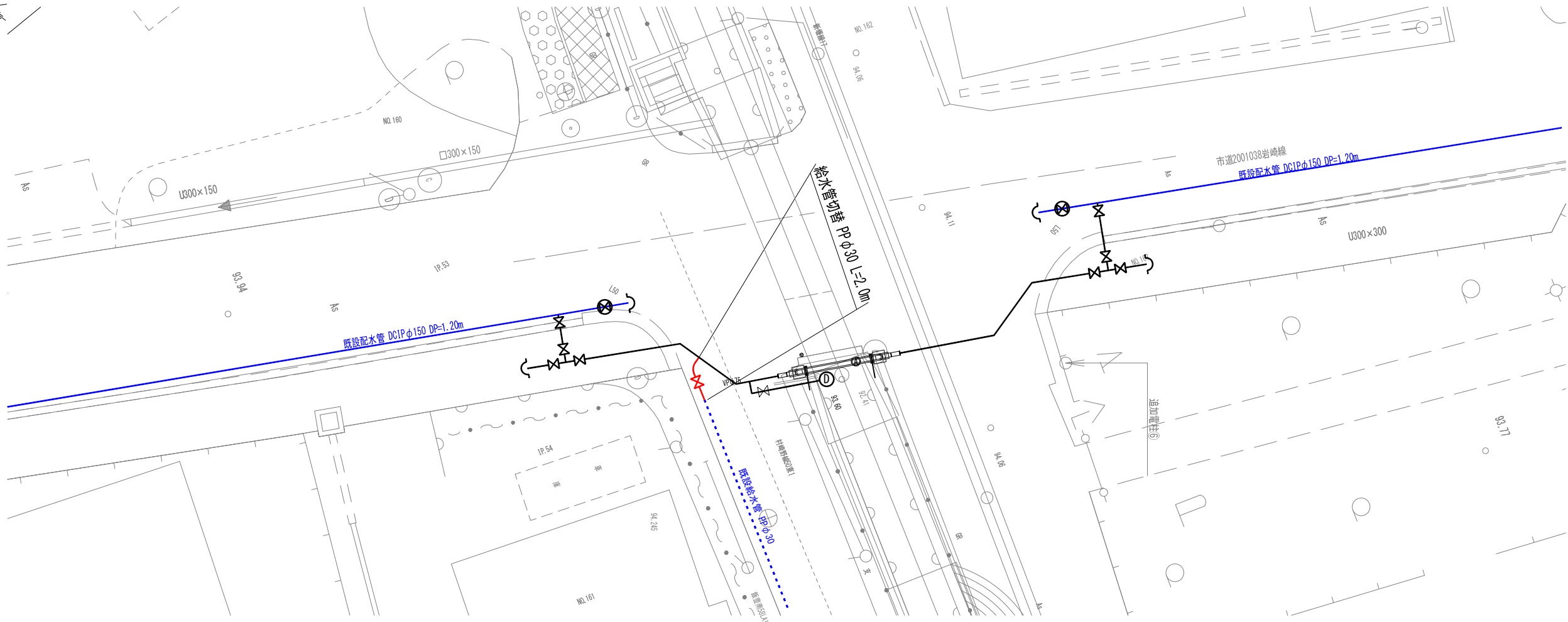
給水管詳細図 NON SCALE
