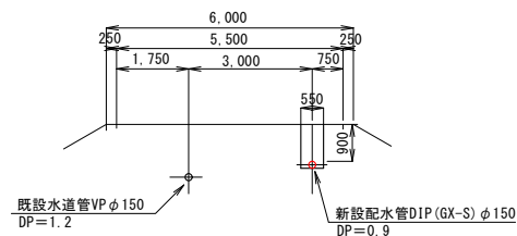
②-②断面図 S=1:100
