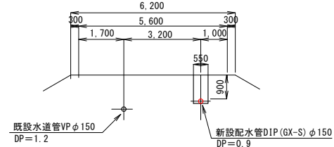
①-①断面図 S=1:100
