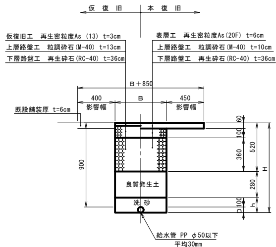
市道車道舗装 (5.0≦W<6.5m) As-2タイプ
