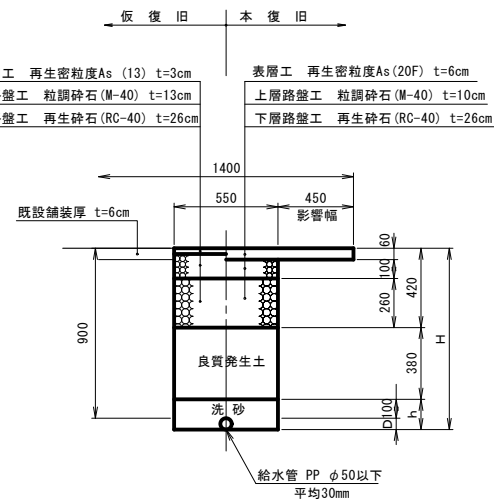
市道車道舗装 (W<5.0m) As-3タイプ
