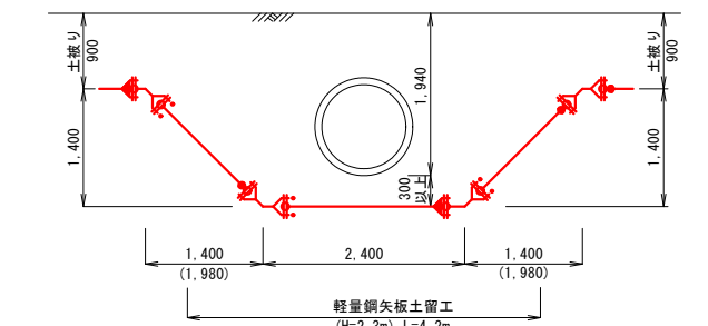
A-A断面
