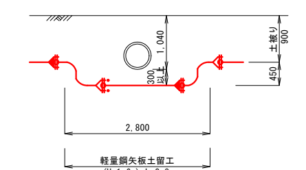
B-B断面
