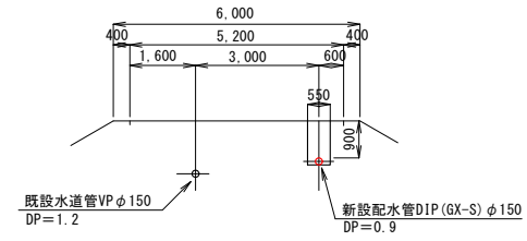
③-③断面図 S=1:100
