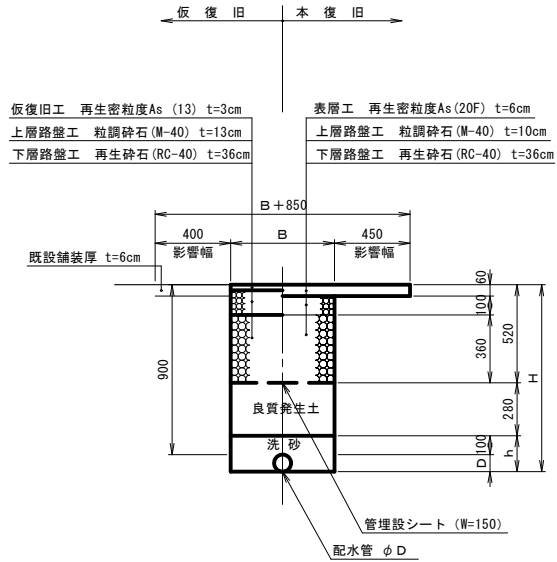
市道車道舗装 (5.0≦W<6.5m) As-2タイプ
