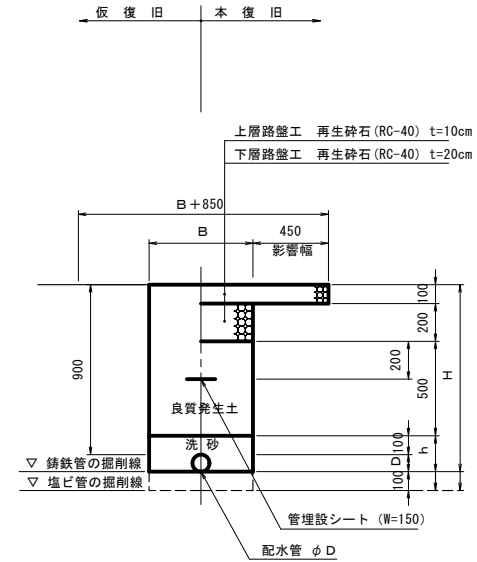
市道砂利道 砂利タイプ
