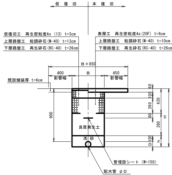
市道車道舗装 (W<5.0m) As-3タイプ
