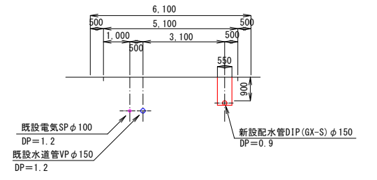
④-④断面図 S=1:100
