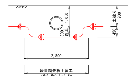
O-O断面 (HPφ500)
