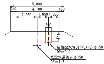
⑥-⑥断面図 S=1:100
