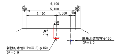
⑨-⑨断面図 S=1:100
