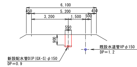
⑧-⑧断面図 S=1:100
