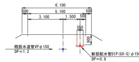
⑦-⑦断面図 S=1:100
