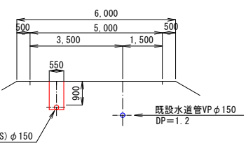
⑫-⑫断面図 S=1:100
