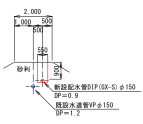
⑪-⑪断面図 S=1:100
