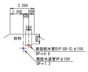
⑪-⑪断面図 S=1:100
