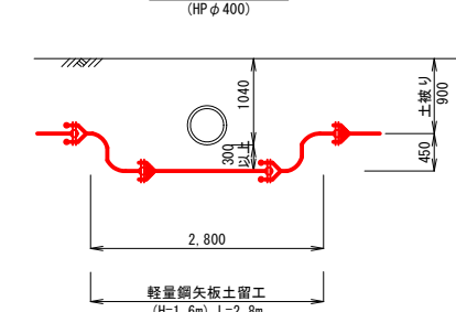
L-L断面
