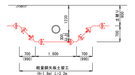
M-M断面 (HPφ300)
