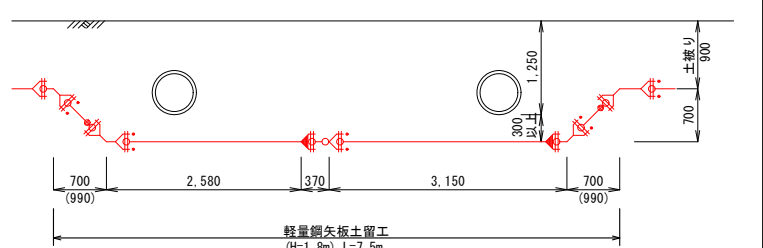
N-N断面 (HPφ500)
