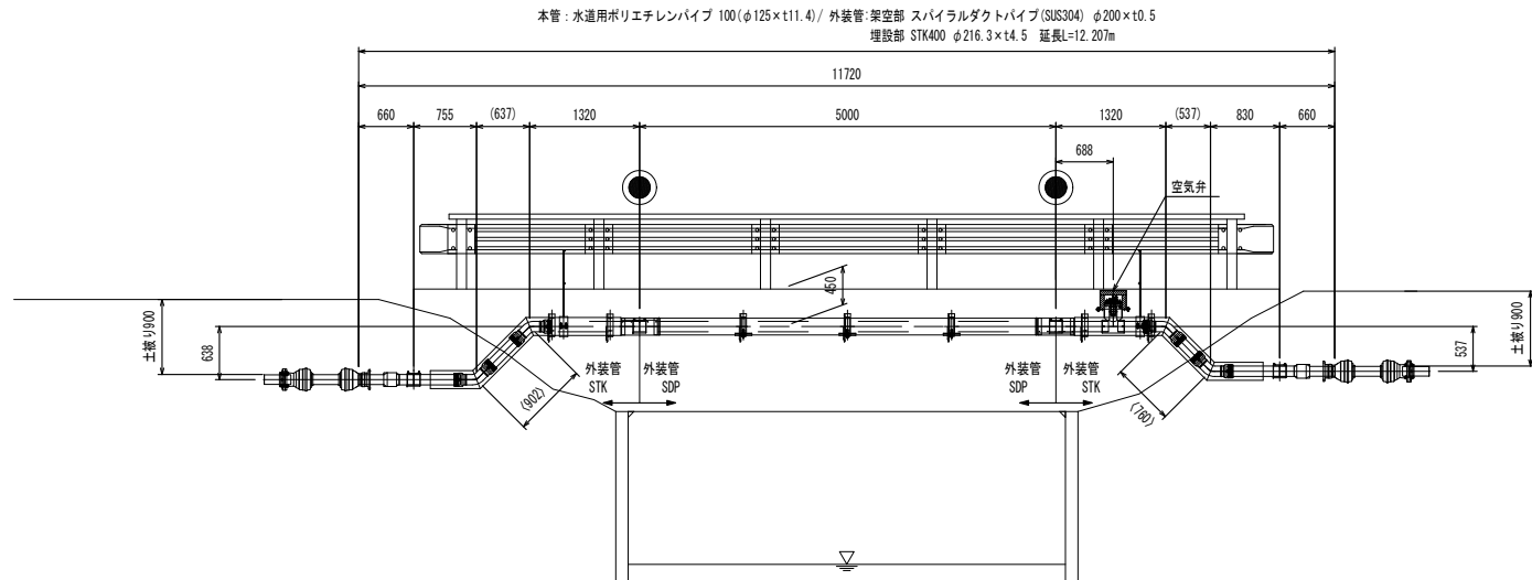
側面図 S=1:50
