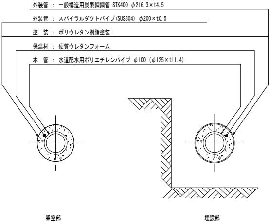
二重管保温工図
