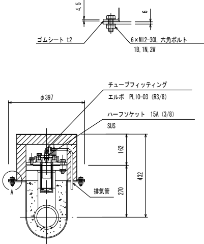
カバー A 詳細
