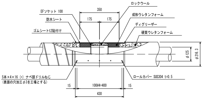
管接続部 (SDP+STK) S=1:10
