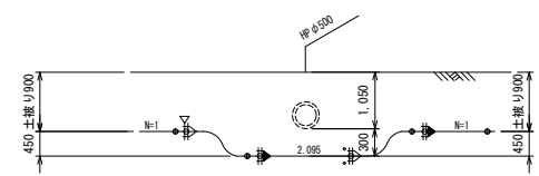
B - B 断面 土留工 H=2.0m L=3.9m
