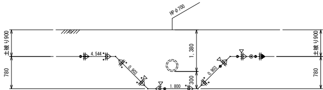
A - A 断面 土留工 H=2.0m L=3.6m
