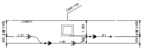
A - A 断面 土留工 H=2.0m L=3.7m
