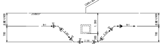
B - B 断面 土留工 H=2.0m L=3.7m
