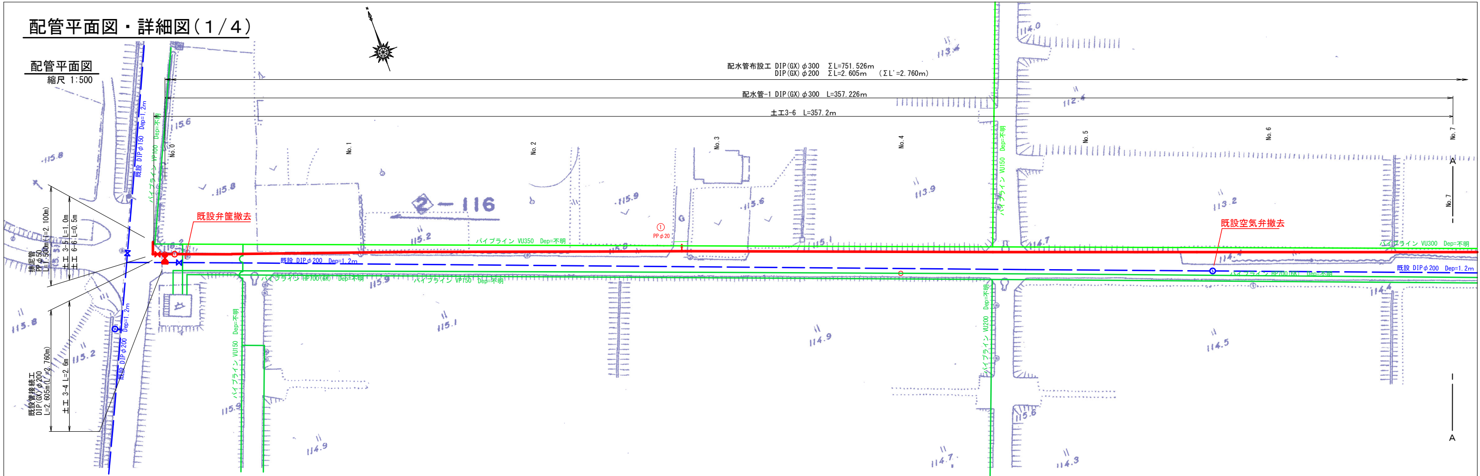
配管詳細図 S-Free
