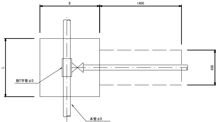
土工⑮ (As-1タイプ) 平面図
