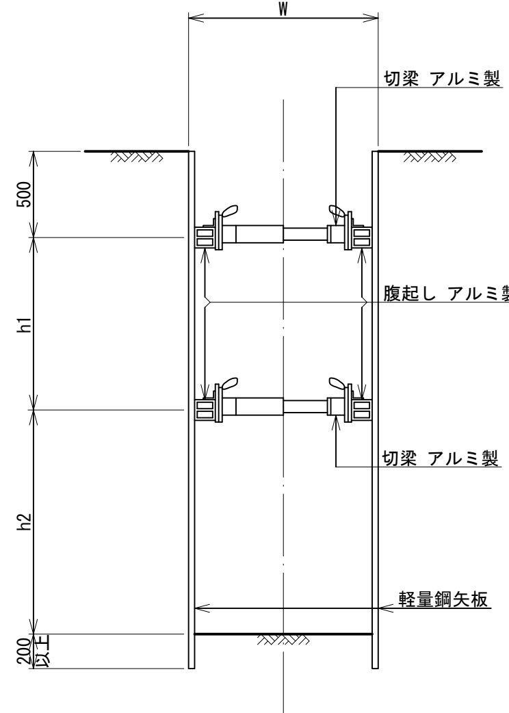
二段支保断面図 (2.0m < 掘削深 ≦ 3.5m)
