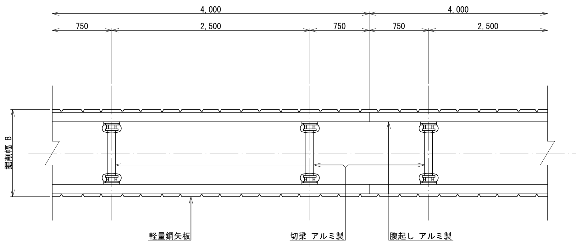
一段支保断面図 (掘削深≦2.0m)
