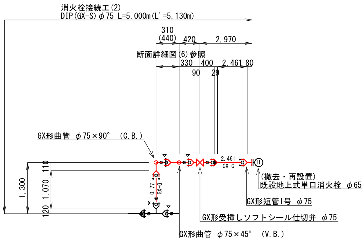
消火栓接続工(2)
