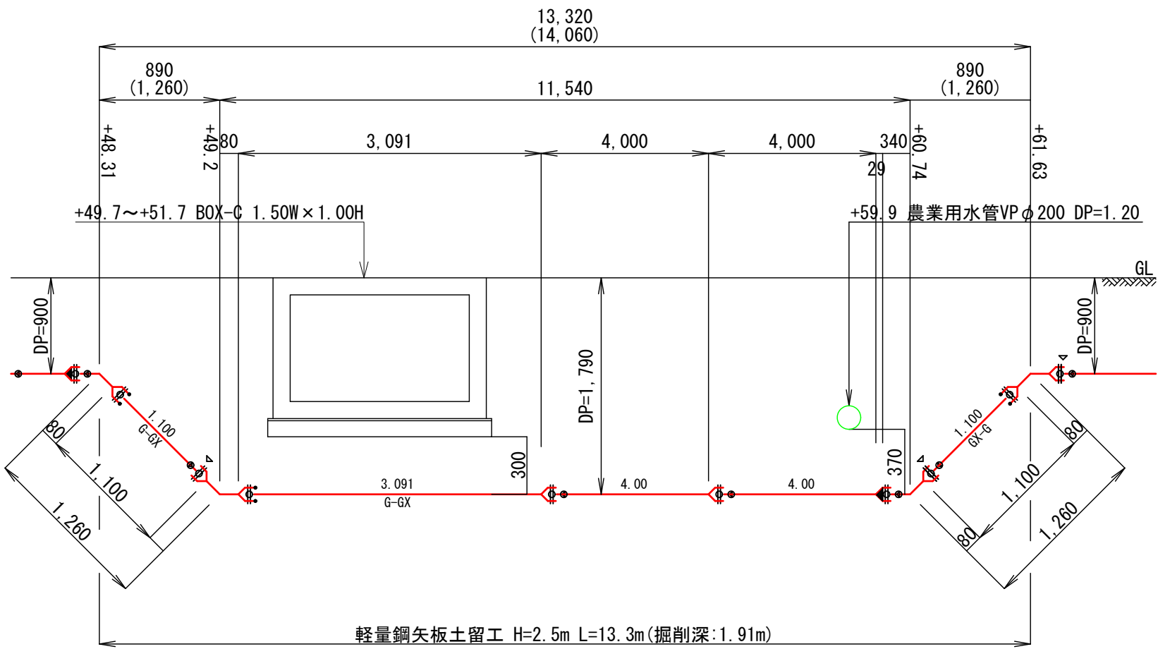
断面詳細図(4)
