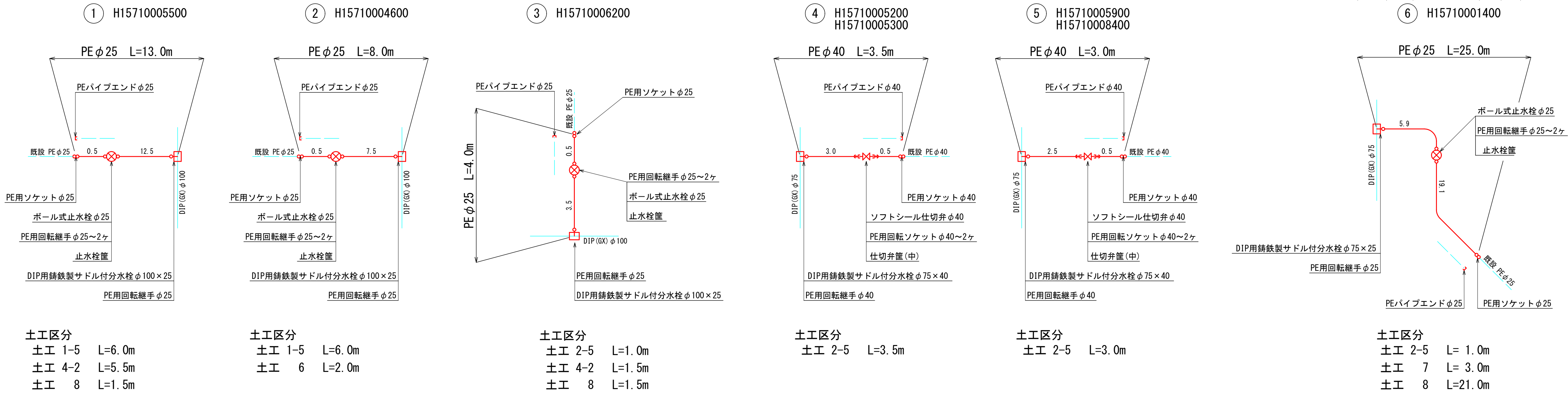
給水管詳細図(1) S=NON SCALE
