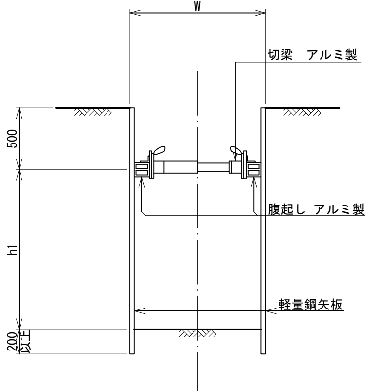
一段支保断面図 (掘削深≦2.0m)
