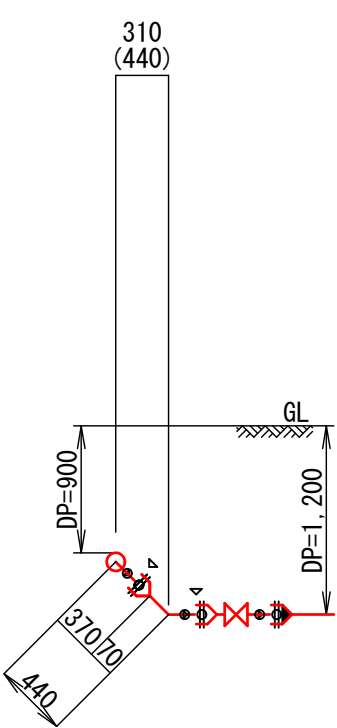
断面詳細図(6)
