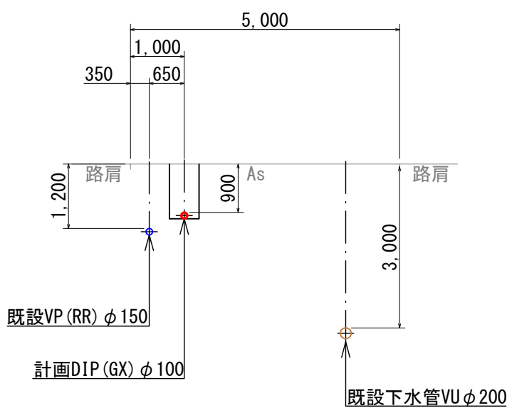
④-④断面図
