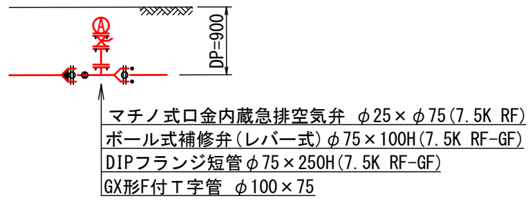
空気弁設置工詳細図 N=1箇所
