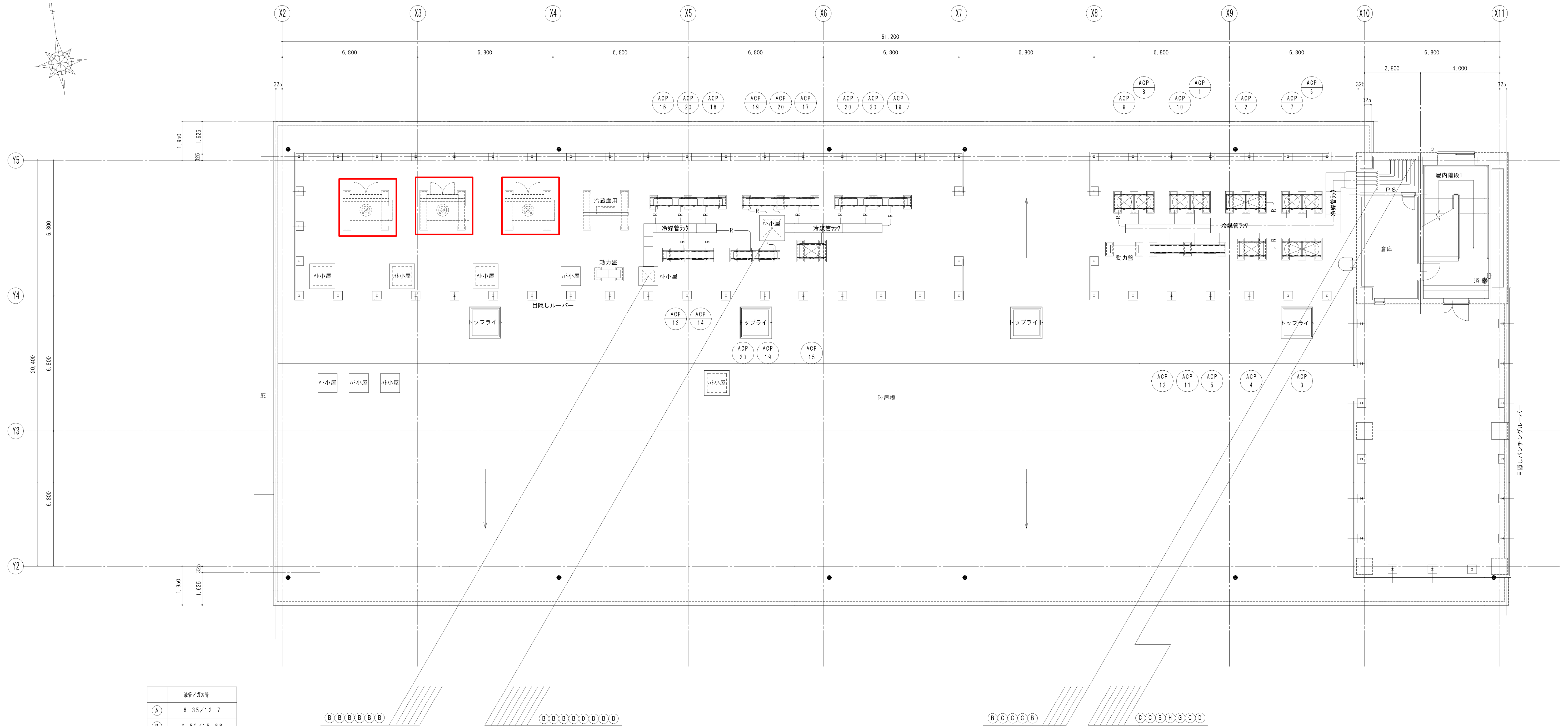
3階平面図 S=1/100 [S=1/200]
